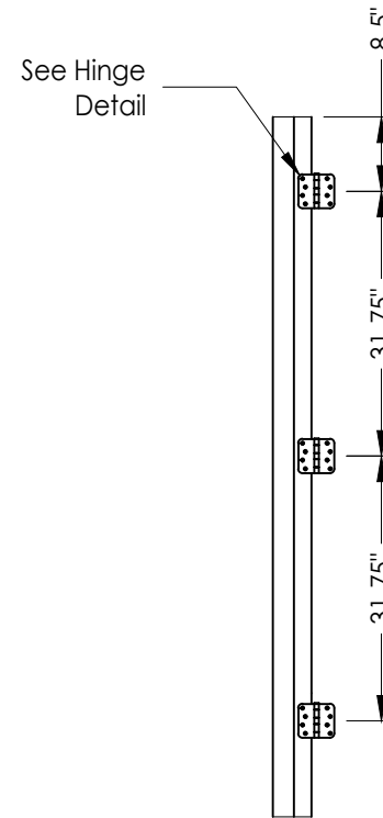
HINGE JAMB
