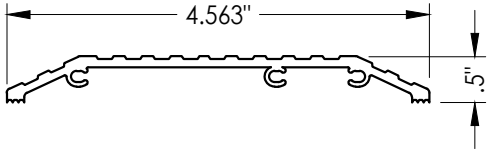
71 ADA SILL
